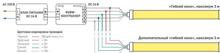
Схема 1. Подключение «гибкого неона» с использованием 4-канального RGBW-контроллера с возможностью изменения цвета свечения и яркости
