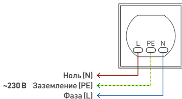
Рис.1. Схема подключения
