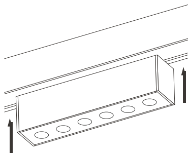
Рис. 2. Установка светильника
