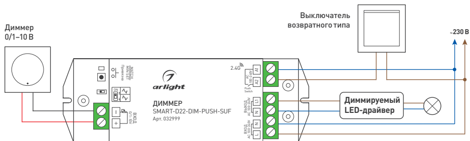
Рисунок 1. Схема подключения диммера SMART-D22-DIM-PUSH-SUF
