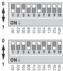
Рис. 2. DIP-переключатели
